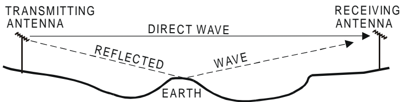
Figure 2-6. VHF LOS.
